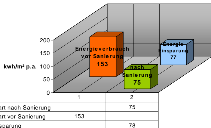
Gegenüberstellung des Wärmeenergiebedarfs (Energiekennzahl) zw. HS Oberwart vorher und nach Sanierung
